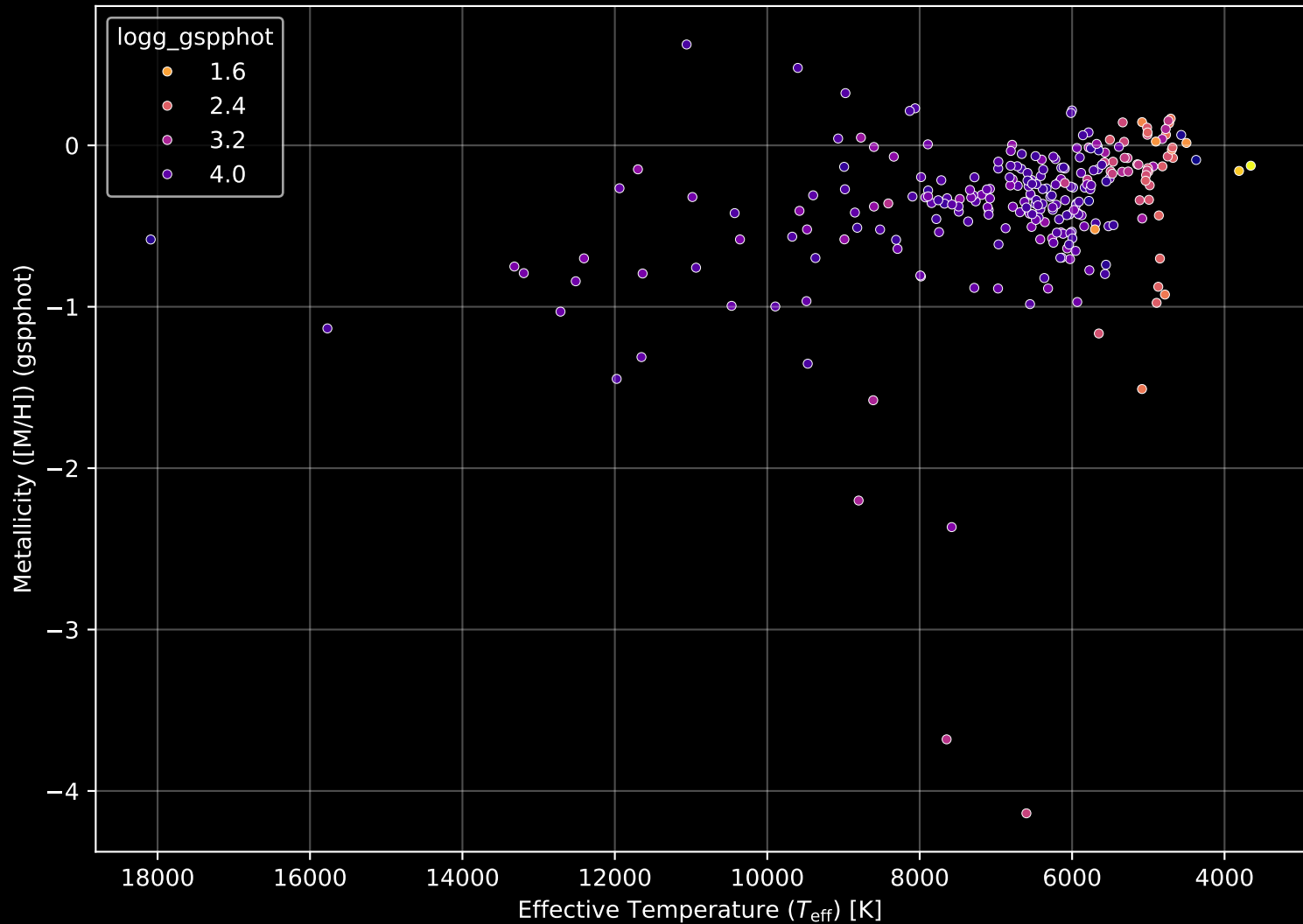
GALAH DR4 Field: [9277] Stellar Population Parameters (n= 258)
